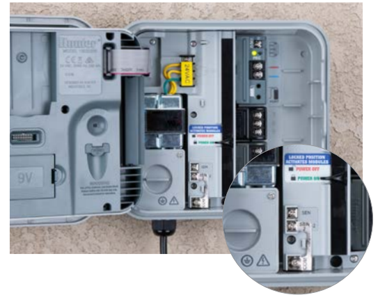
带有 2 个传感器输入端的 P2C-400 控制器
